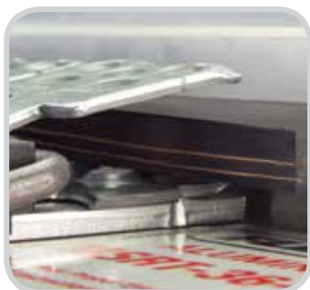
Die abgestufte Bandzuführung erleichtert das Einführen des Transportbandes in den Verbinderstreifen.
